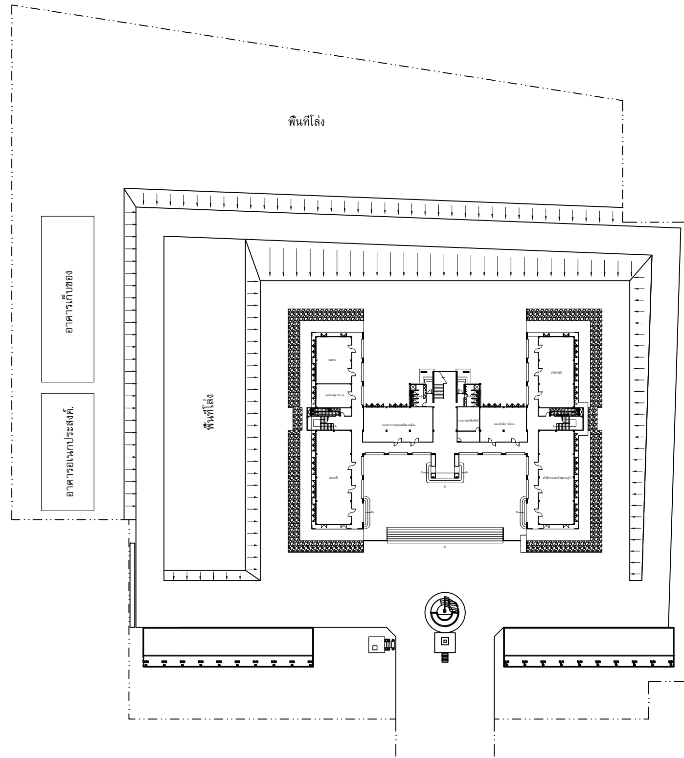
ผังบริเวณอาคารสำนักงานเทศบาลเมืองปากช่อง มาตราส่วน 1:750
